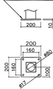
POTEAUX DE RECEPTION AVEC PLATINE À VISSER
