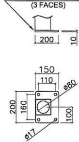
POTEAU DE GUIDAGE AVEC PLATINE À VISSER (3 FACES)
